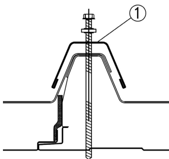
Couvre-joint en tôle pré-peinte
