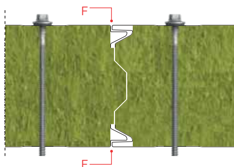
Dettaglio del giunto Tipo 2
