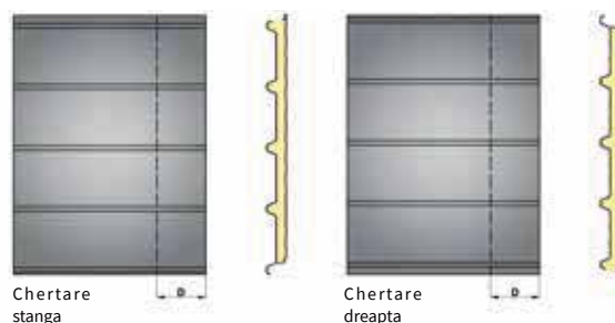
Detaliul sistemului de chertare
